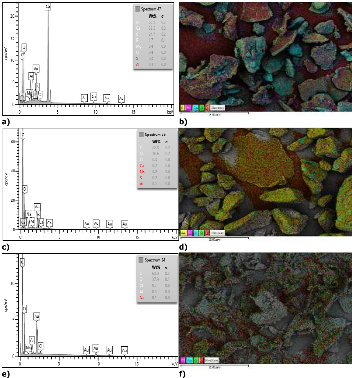
Figura 6. Espectroscopía de energía dispersa ( EDS , en inglés). a), b) Espectros de quitosana mineralizada; c), d) Quitosana obtenida por método convencional; e), f) Quitosana Sigma Aldrich
