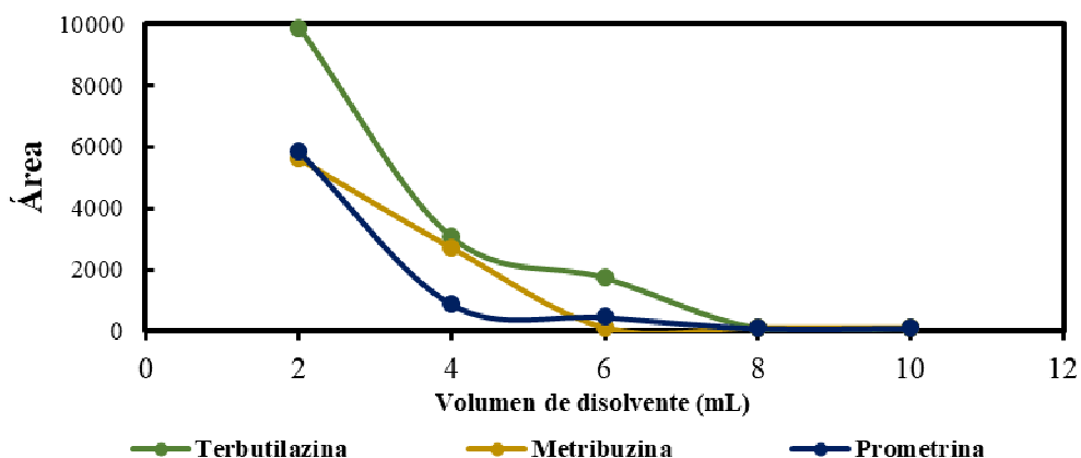
Figura 9. Efecto del volumen de disolvente
