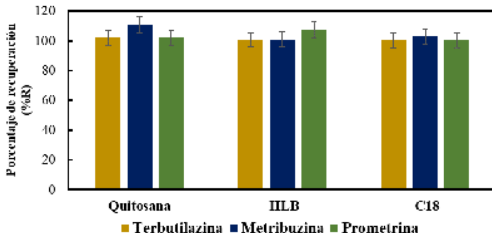
Figura 11. Comparación de la SPE con quitosana obtenida con el sistema MeOH-H 2 O-CaCl 2 y cartuchos comerciales (HLB y C 18 )
