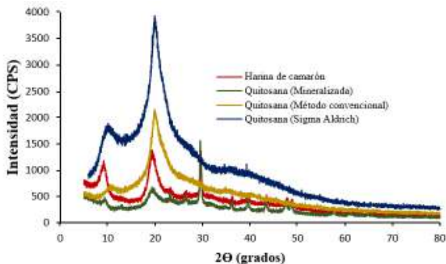
Figura 4. Diffractogramas de harina de camarón, de la quitosana obtenida por método convencional (QNaOH), quitosana mineralizada (QM) y quitosana Sigma-Aldrich (QS)
