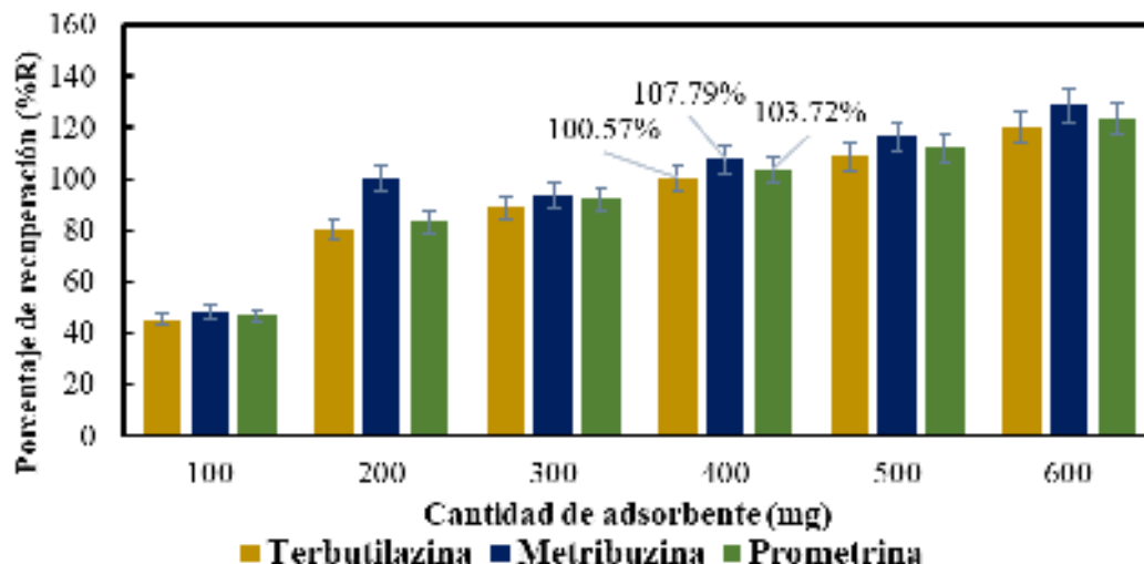
Figura 10. Porcentaje de recuperación debida a la variación en la cantidad de adsorbente
