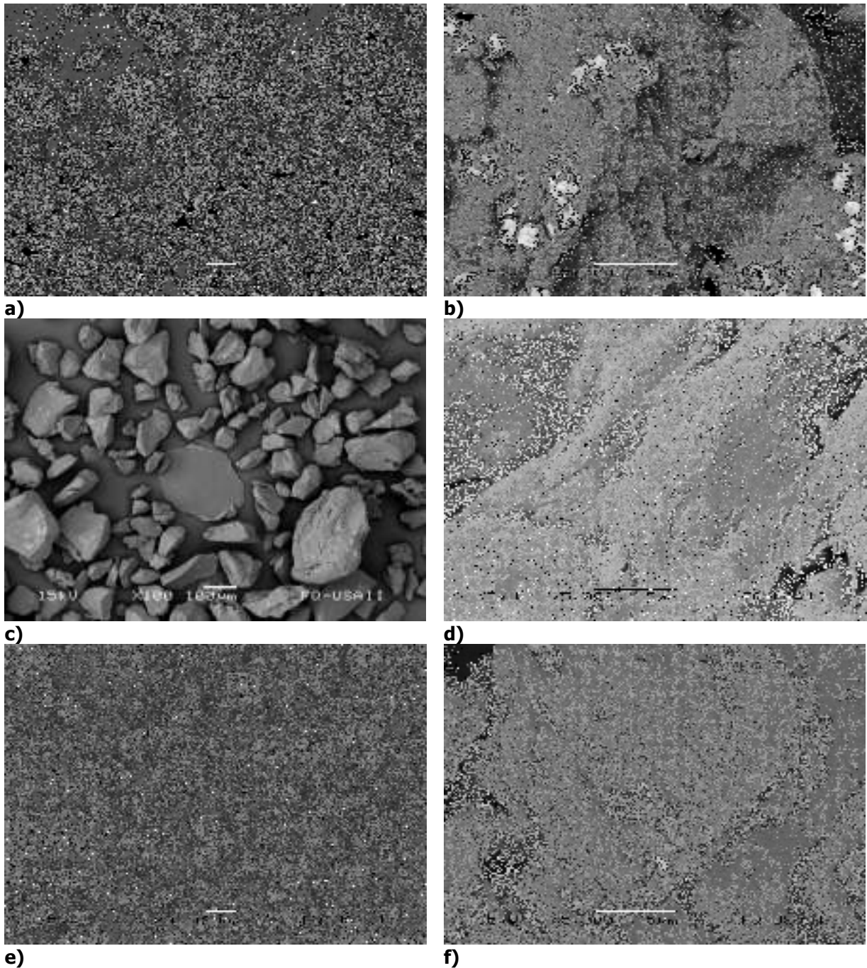
Figura 5. Microscopía electrónica de barrido (SEM, en inglés): a), b) Quitosana mineralizada a 100x y 5000x, respectivamente; c), d) Quitosana obtenida por método convencional a 100x y 5000x, respectivamente; e), f) Quitosana Sigma Aldrich convencional a 100x y 5000x, respectivamente
